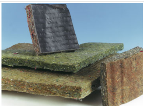
Mit Phenolharz gebundene Baumwollvliese, teilweise mit Schwerschicht Phenolic Resin-Bonded Cotton Webs, Partially with a Heavy Layer
